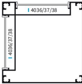
4003 Stub za ogradu 50x50 S 50x50x1,6 mm
