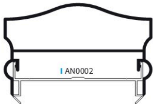
AN0001 Rukohvat ANTICK 130x80x1,4 mm
