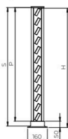
Presjek A-A ispuna 60x20
