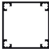
4006 Stub za ogradu 75x75 75x75x1,6 mm
