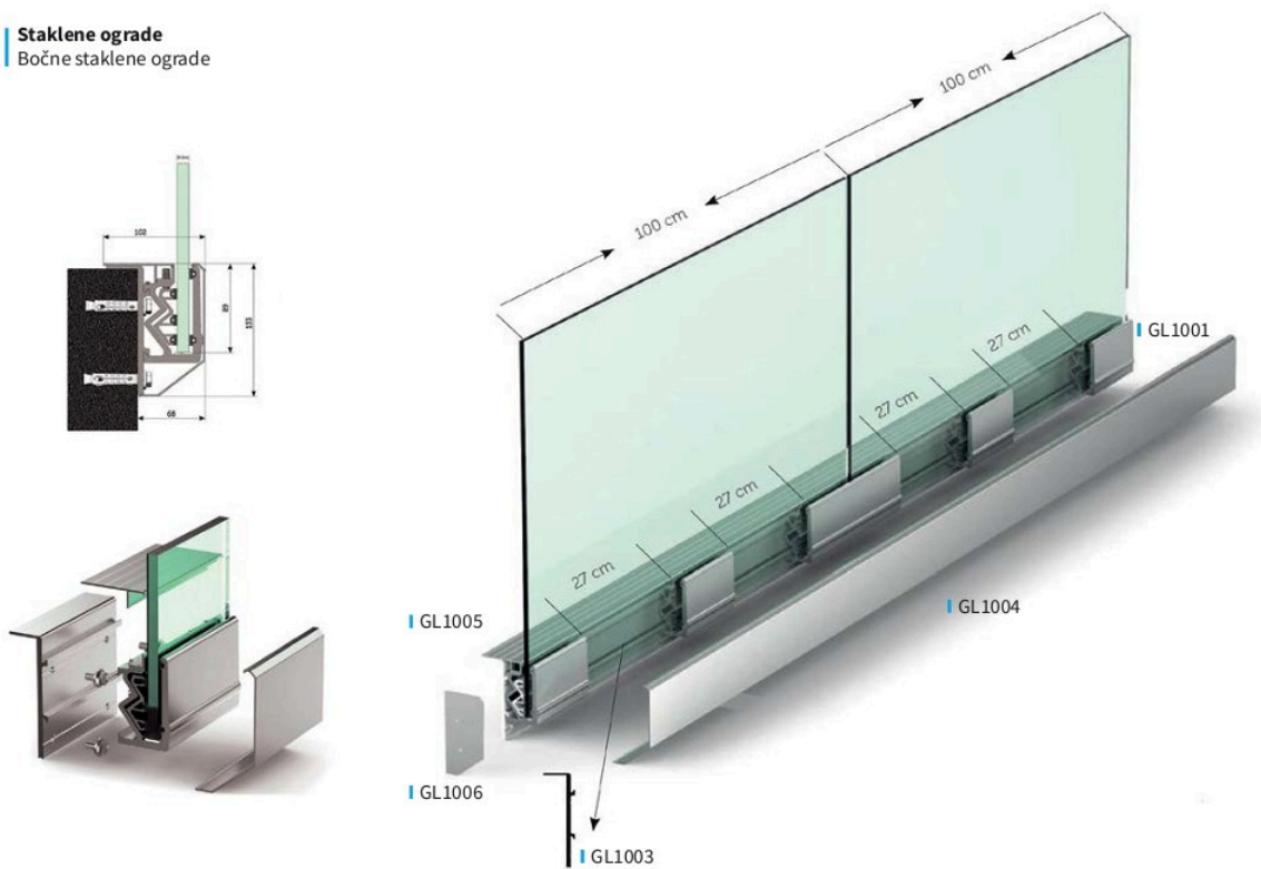
GL1001 Nosač 15 cm za bočnu staklenu ogradu za staklo 12-15 mm
